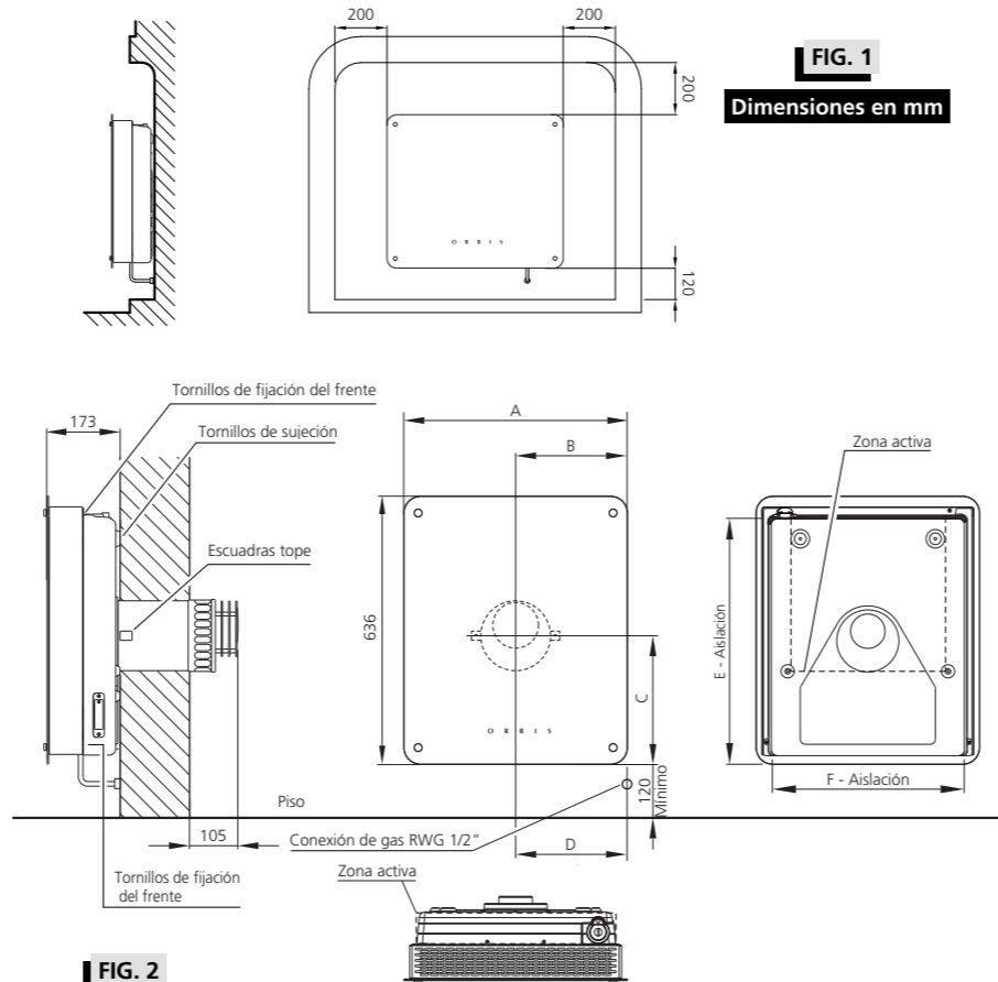
FIG. 2 Dimensiones en mm
